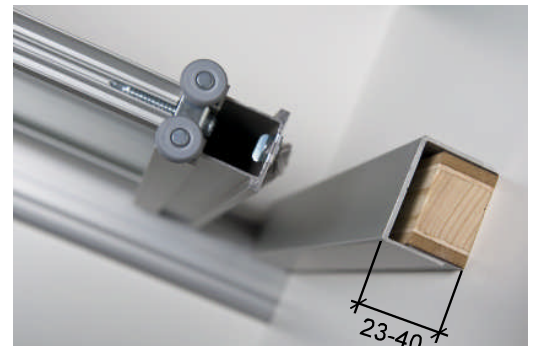
Abb. 2 Aufschieben des Klemmprofils
