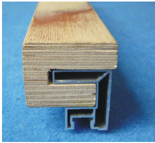
Abb. 1 slide quattro asymmetrisch
